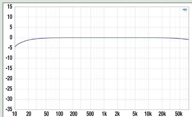
Linearer Frequenzgang bis weit über 50 kHz. Damit eignet sich der CVR-200 auch bestens für HiRes-Musik mit Superhochton-Anteil.
