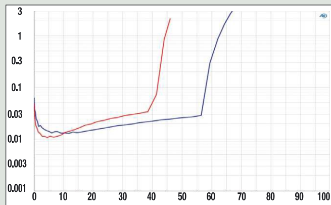
Sowohl an 8 als auch an 4 Ohm zeigt der Block sauberes Klirrverhalten bis zur Leistungsgrenze.
